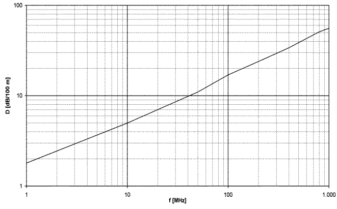
Dämpfungsverlauf
